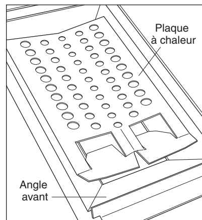
Plaque rayonnante du gril type charbon de bois
