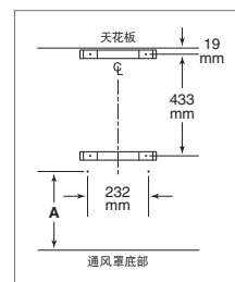
安装位置。
