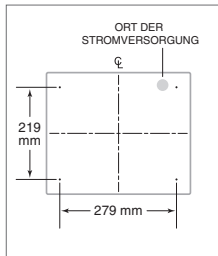
Montageort
