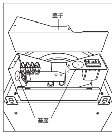
接线位置。
