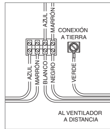
Cables del ventilador a distancia.
