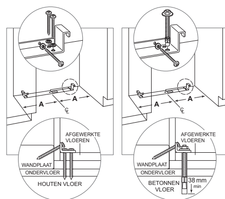
Houten vloer
