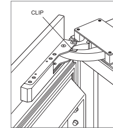
90° door stop
