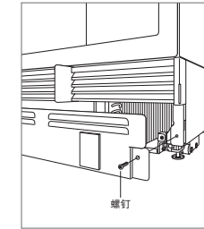
踢脚板拆卸
