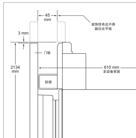
上部窗框 (侧视图)
