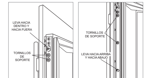
Ajuste hacia dentro y hacia fuera
