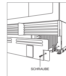
Ausbauen der Sockelleiste
