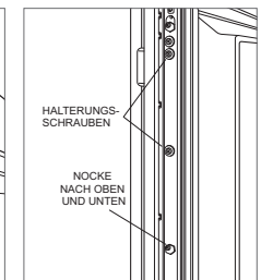
Anpassung nach oben und unten
