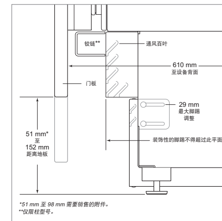
脚踏 (侧视图)
