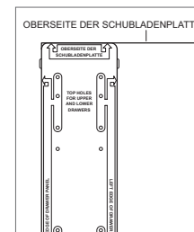
Schubladenplattenvorlage - oben
