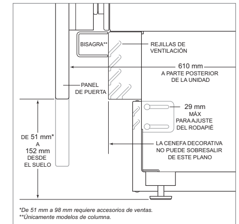
Rodapié (vista lateral)
