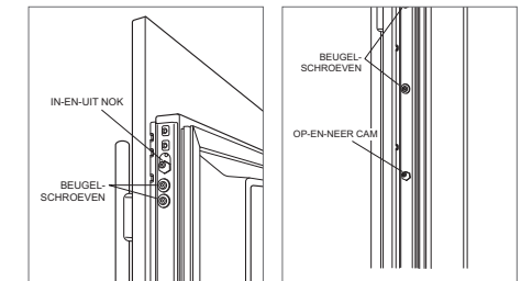
Aanpassing in-en-uit
