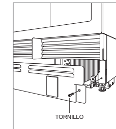
Extracción del zócalo
