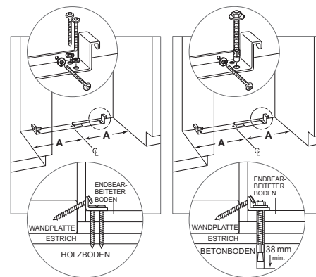
Holzboden
