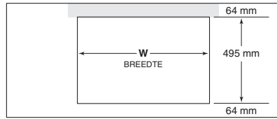
UITSPARING AANRECHT
