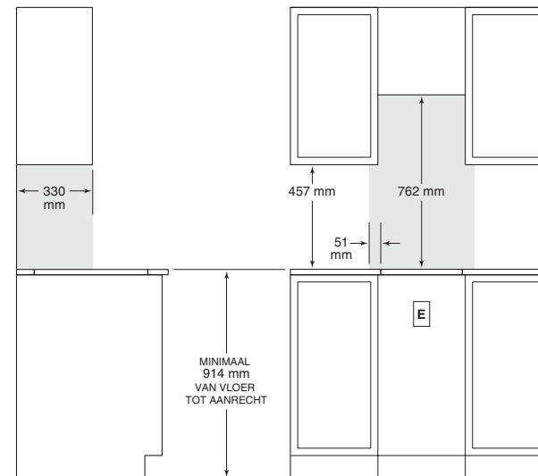
ZIJAAZICHT
