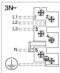
Verdrahtungsdiagramm, 3-phasig
