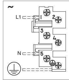
单相接线图
