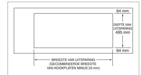
Uitsparing aanrecht
