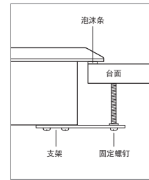
灶具安装
