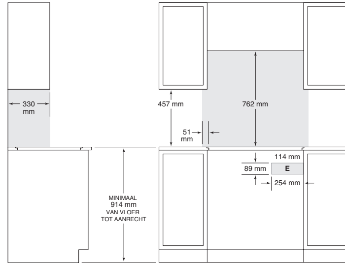
ZIJAAZICHT
