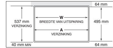
UITSPARING AANRECHT
