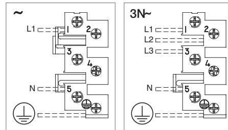
Schéma de câblage monophasé
