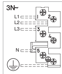
Schema elettrico dell'impianto trifasico
